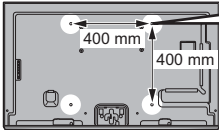
Rückseite des Fernsehers
