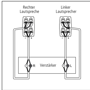
Zweifach-Verkabelung
