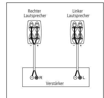
Normale Verkabelung
