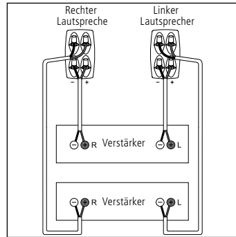
Zweifach-Verstärkung
