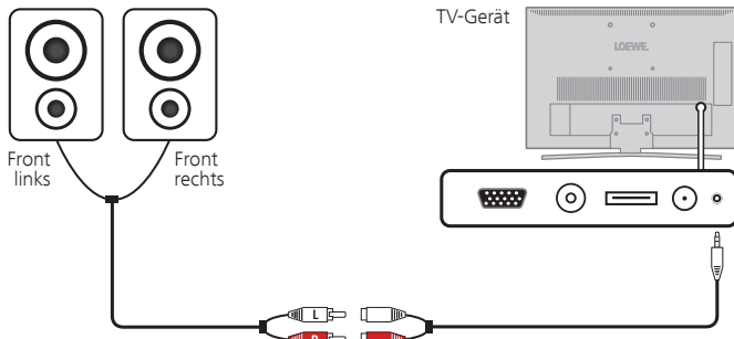
Anschluss von Aktivlautsprechern an das TV-Gerät
