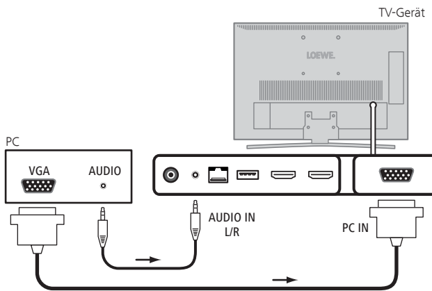
Anschlussbeispiel eines PC
