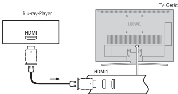
Anschlussbeispiel eines HDMI-Gerätes (z.B. Blu-ray-Player)
