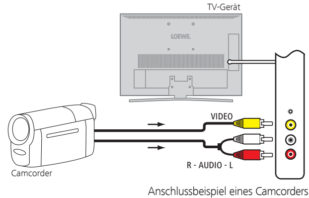
Anschlussbeispiel eines Camcorders
